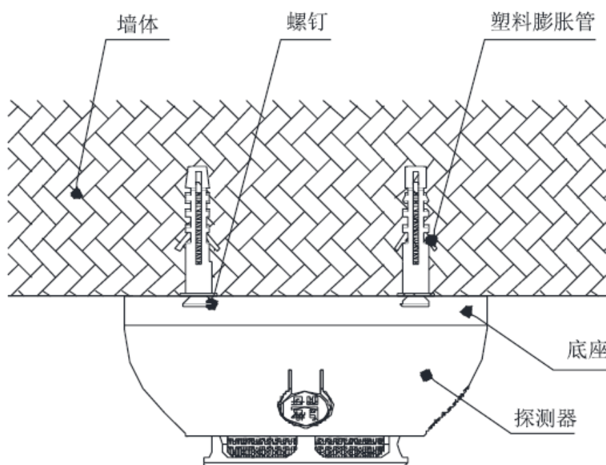
螺钉安装示意图
