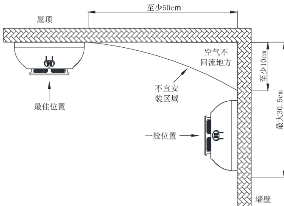
屋顶和墙壁安装位置示意图
